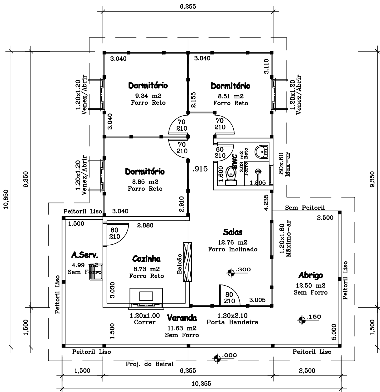
Planta Baixa 87.55 m 2
